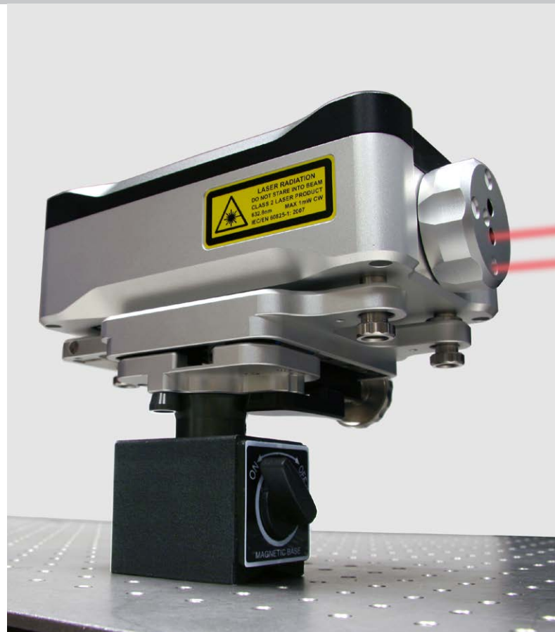
Système à laser XL-80 monté sur socle magnétique
